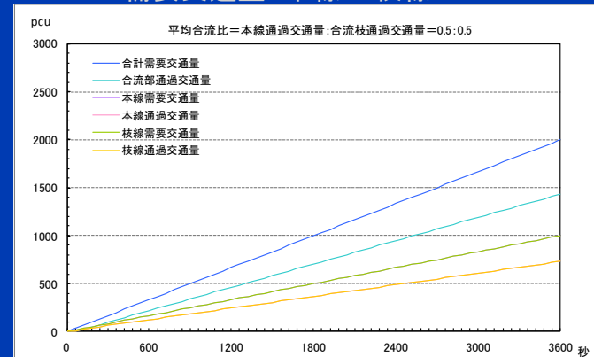
需要交通量 本線5:枝線5
