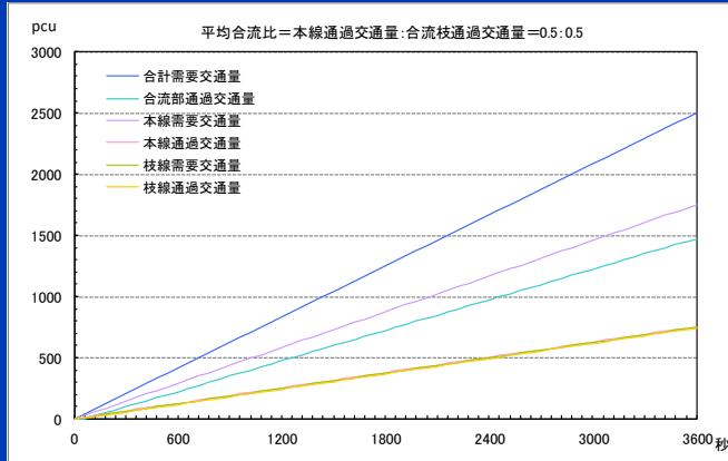
需要交通量 本線7:枝線3
